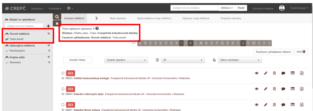
Obrázok 9: Zoznam výsledkov hľadania obsahujúci len tretiu úroveň (katedry) vďaka použitiu fazety Úroveň inštitúcie
